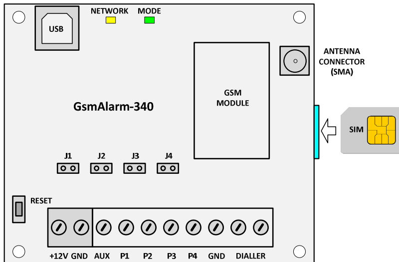
Контакты соединения и световые индикаторы модуля GsmAlarm-340
