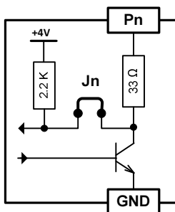
Эквивалентная схема P1 - P4
