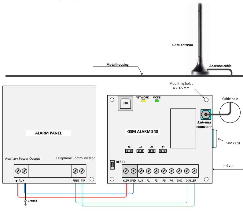
Схема соединения модуля GsmAlarm-340
