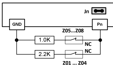
ATZ mode (A4Y)
